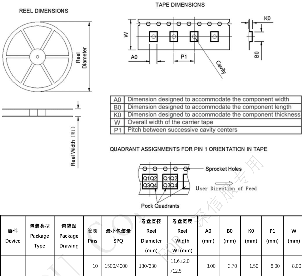
图 5 包装图
