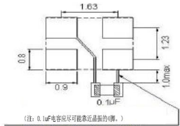
推荐焊盘尺寸 (mm)
