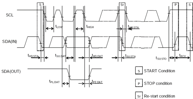
图 22 I 2 C 时序图
