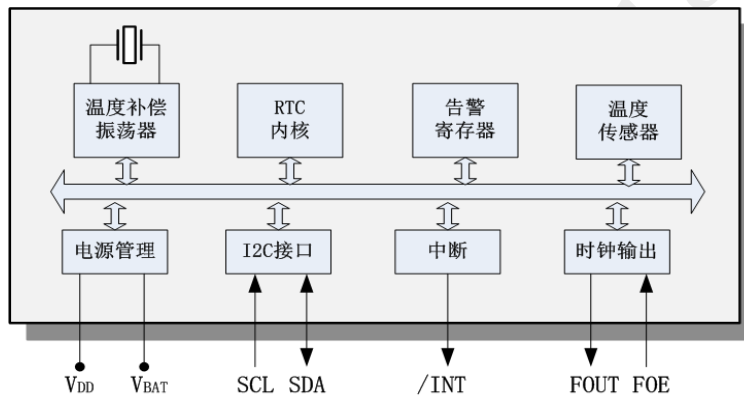
图 1-1 原理框图
