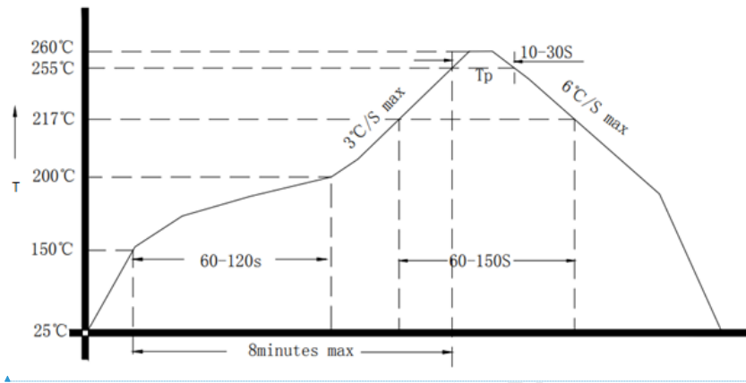
图 33 封装焊接曲线
