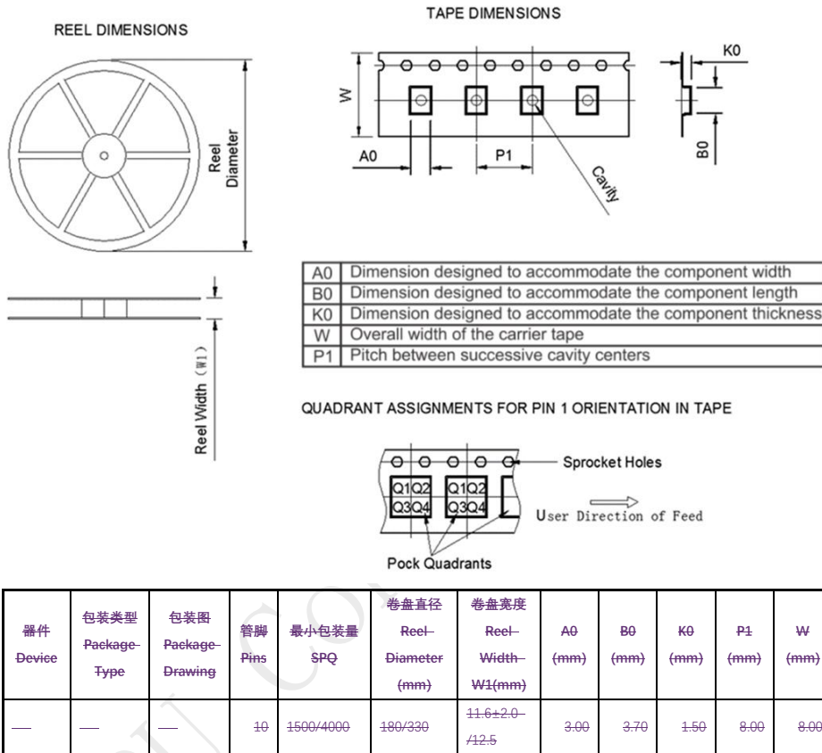
图 4 封装尺寸及推荐焊盘
