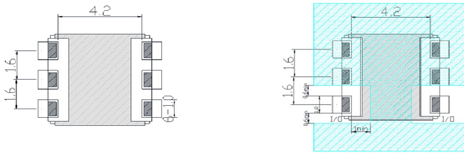
DIMENSION UNIT:mm
