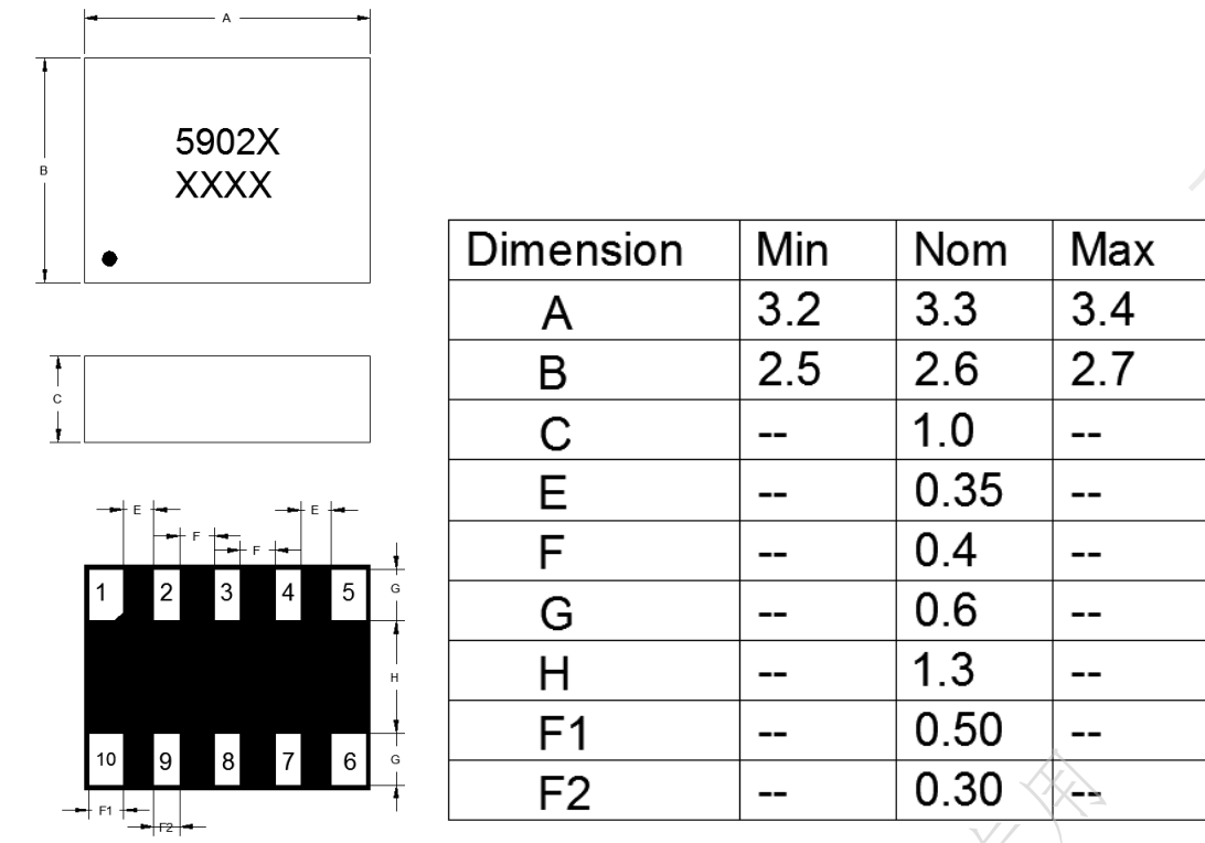
图 4 封装图
