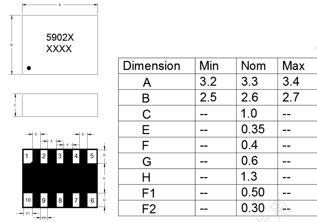
图 4 封装图
