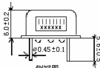
侧视图
