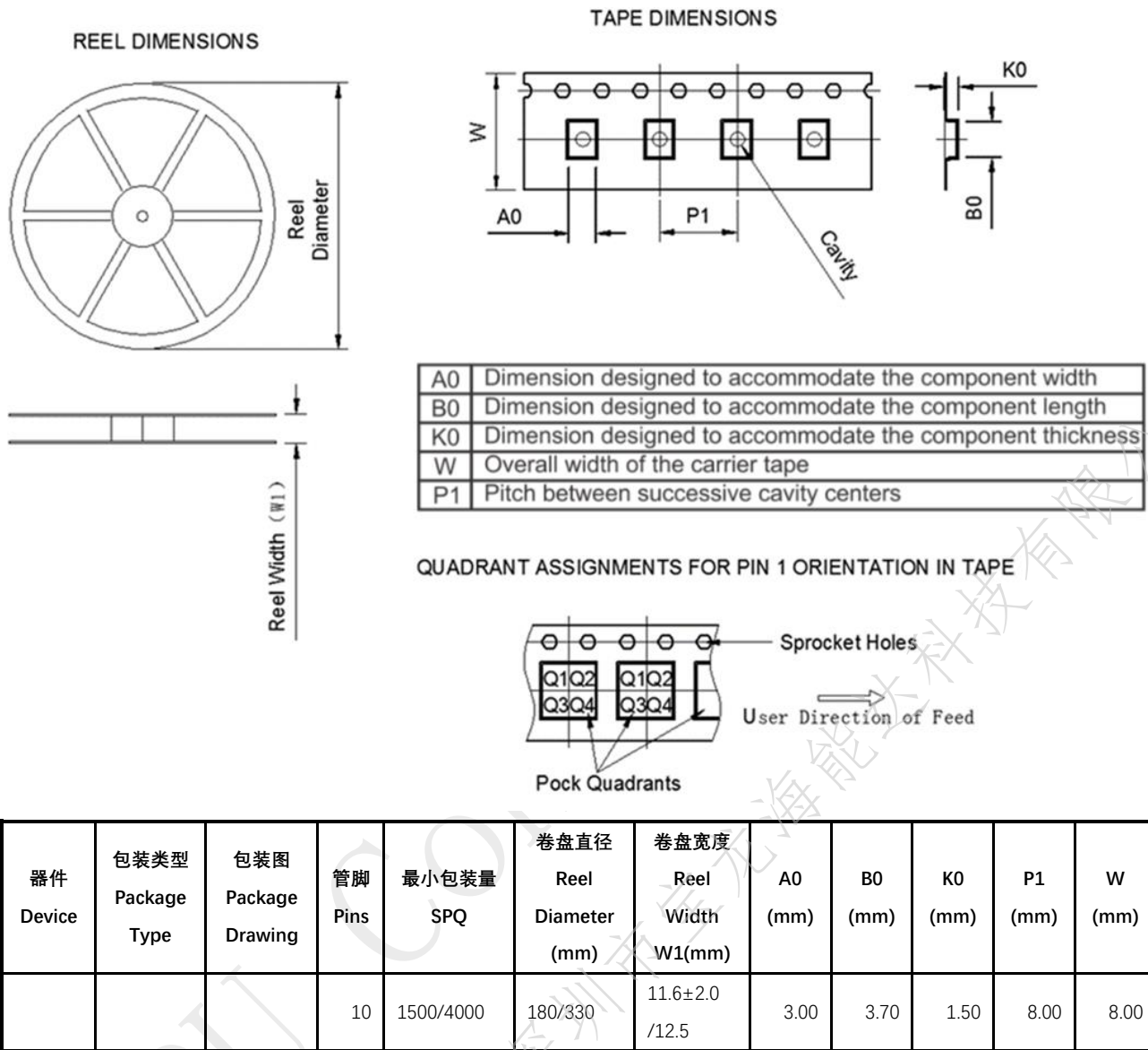
图 5 包装图
