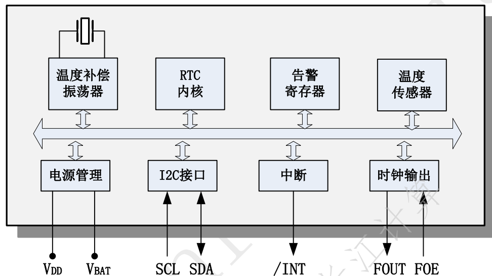
图 1 原理框图
