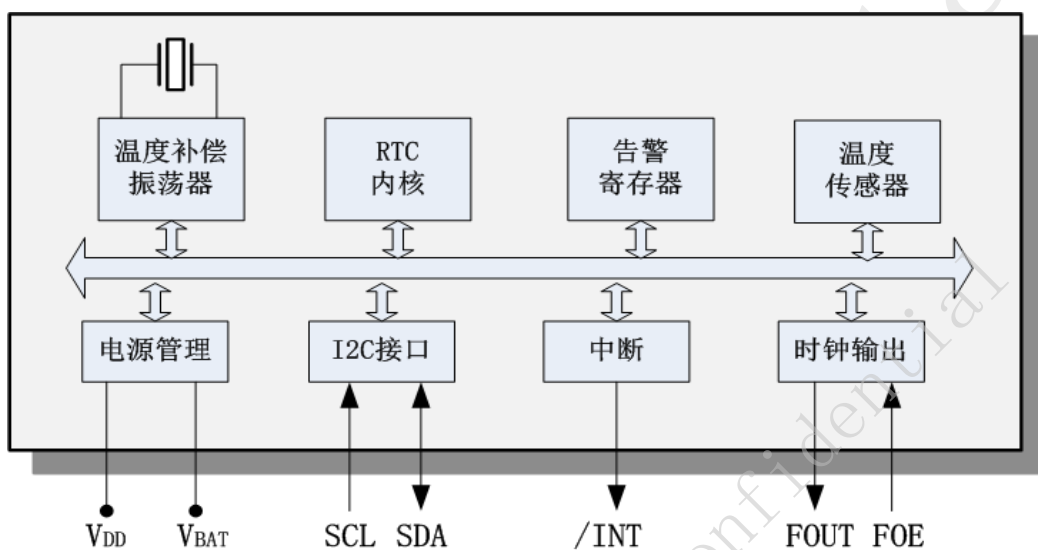
图 1 原理框图
