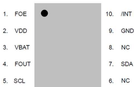
图 2 管脚分布图
