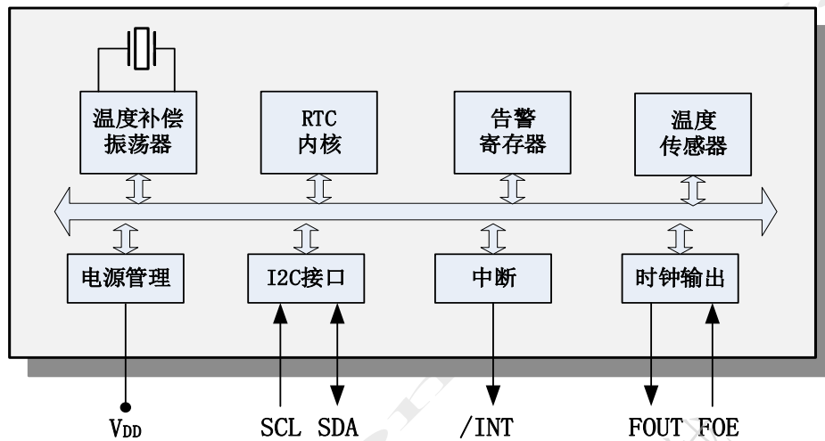
图 1 原理框图
