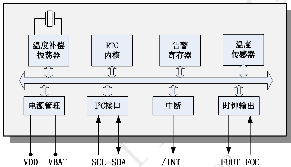
图 1 原理框图
