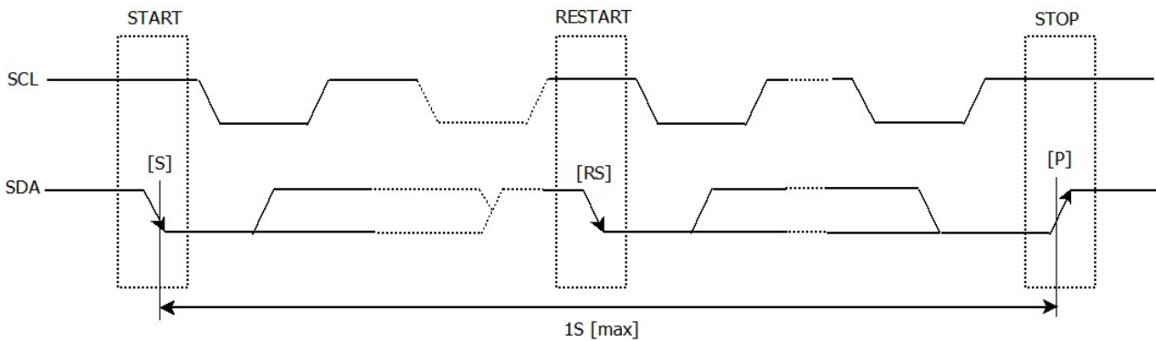
图 5 I 2 C 总线接口
