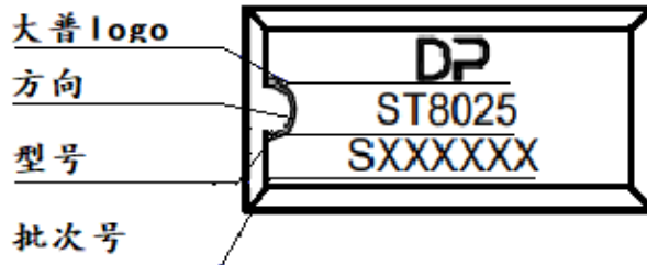
图 5 丝印信息
