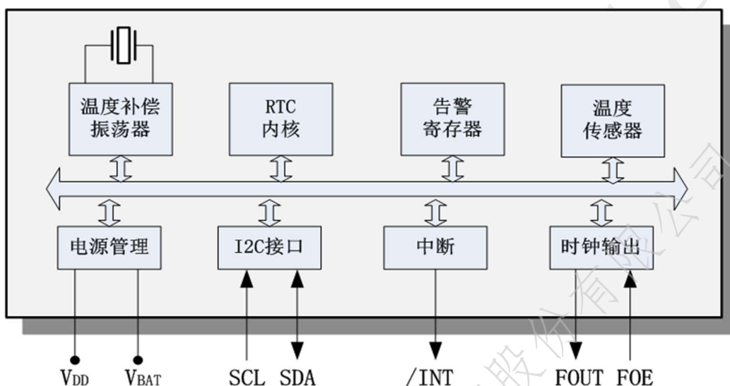
图 1 原理框图
