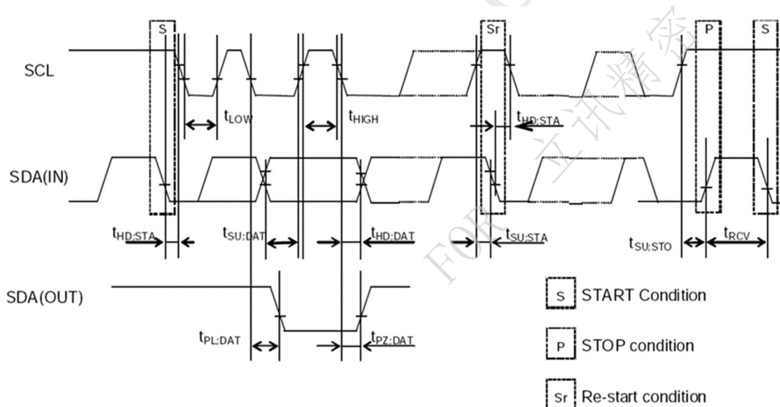
图 2 I 2 C 时序图
