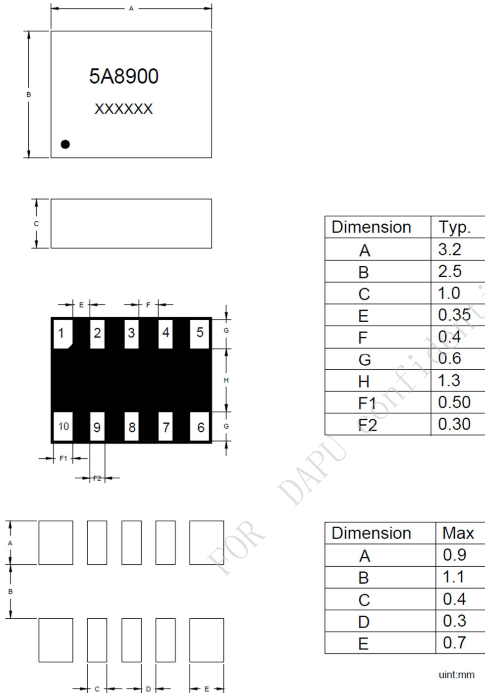
图 4 封装尺寸及推荐焊盘
