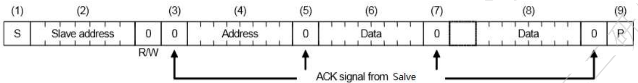
图 6 写序列
