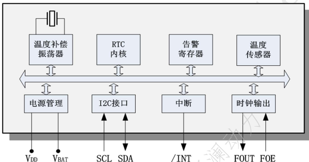
图 1 原理框图
