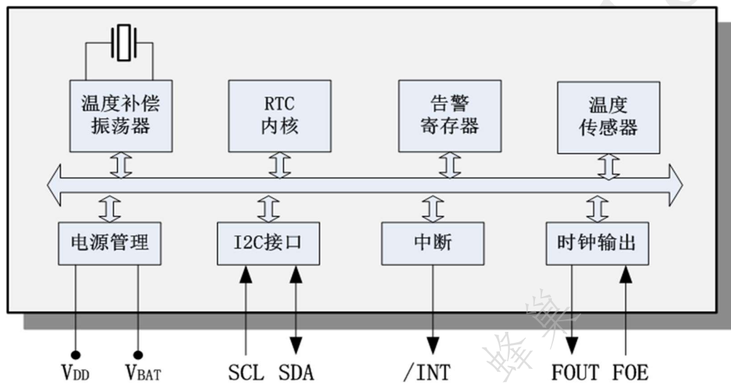
图 1 原理框图
