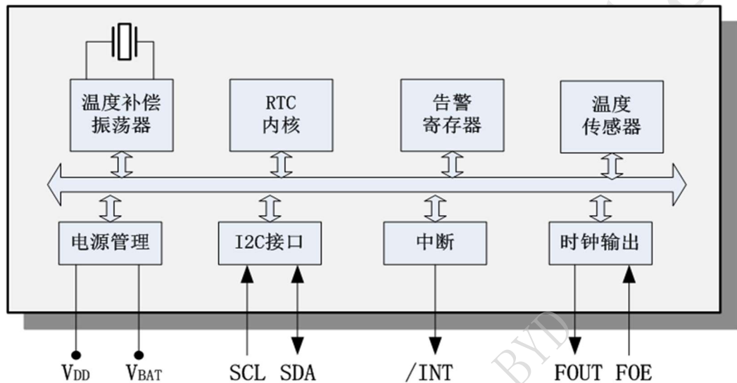
图 1 原理框图
