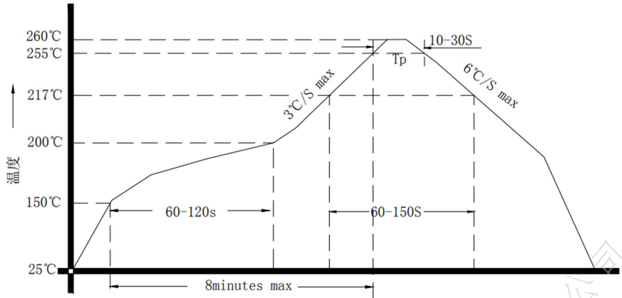
图 10 回流焊曲线
