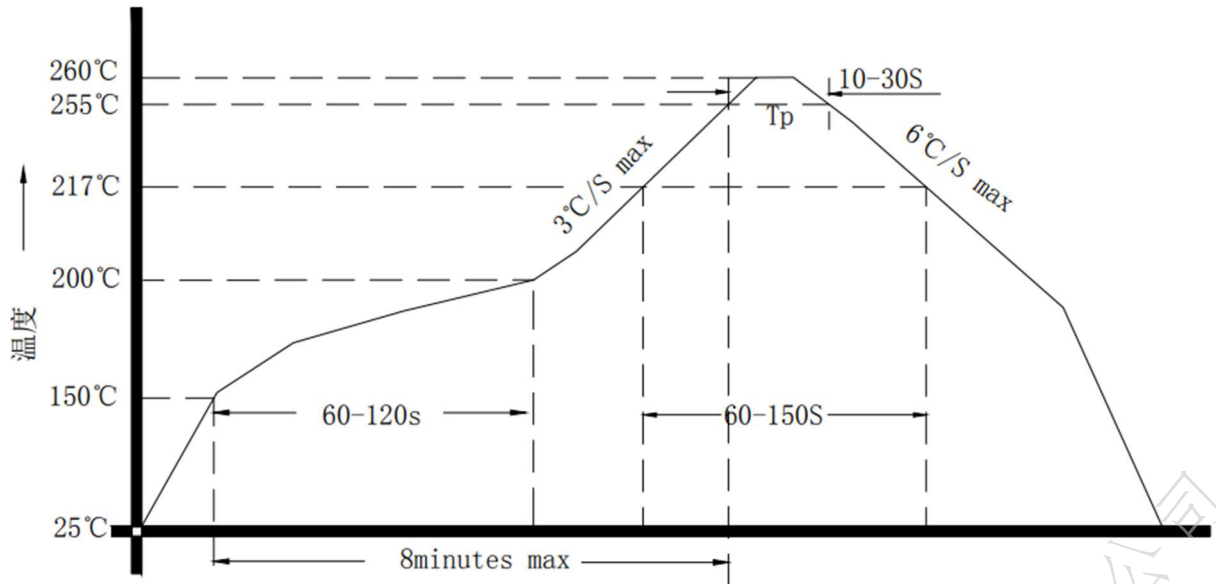
图 10 回流焊曲线
