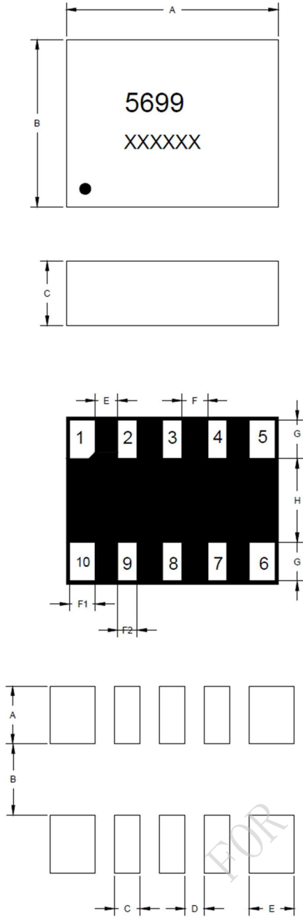
图 4 封装尺寸及推荐焊盘
