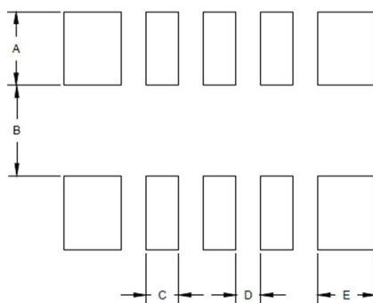
图 4 封装尺寸及推荐焊盘
