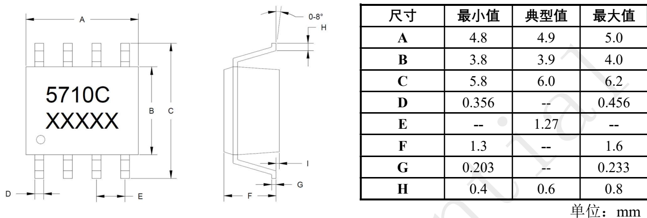
图 3 封装图
