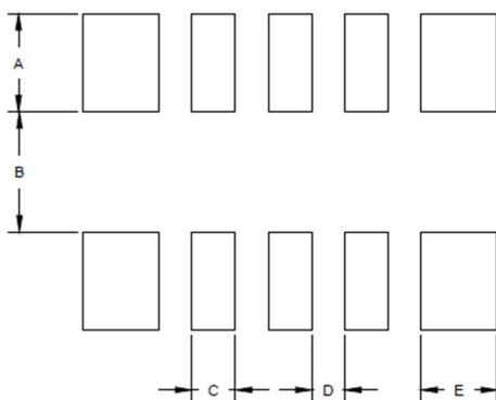
图 4 封装尺寸及推荐焊盘
