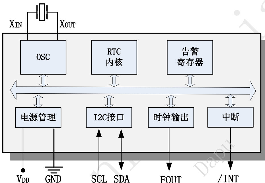
图 1 原理框图
