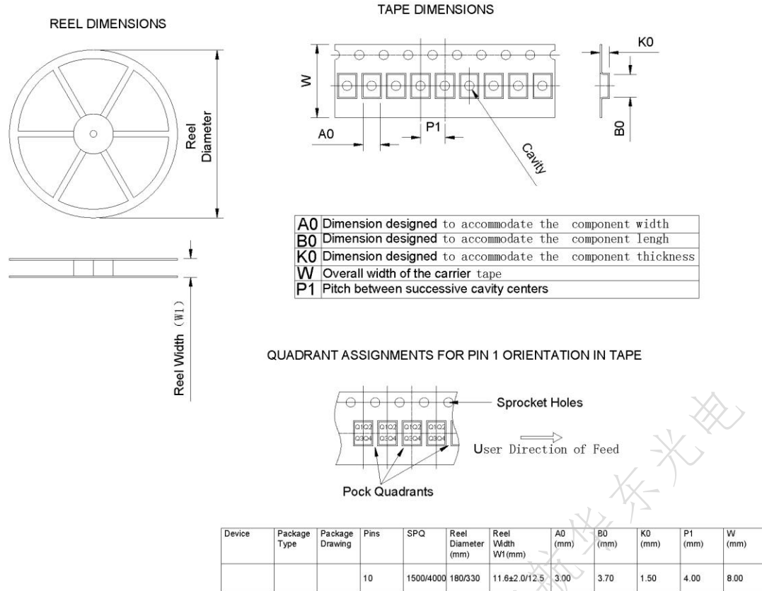
图 11 包装图
