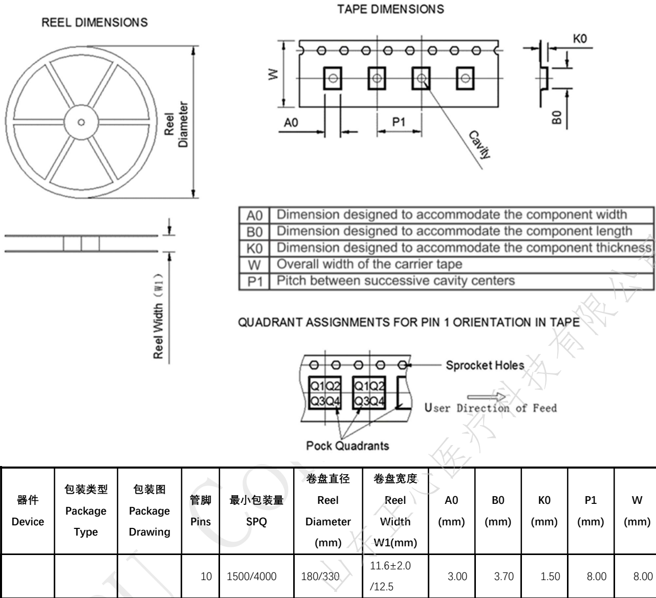
图 6 包装图
