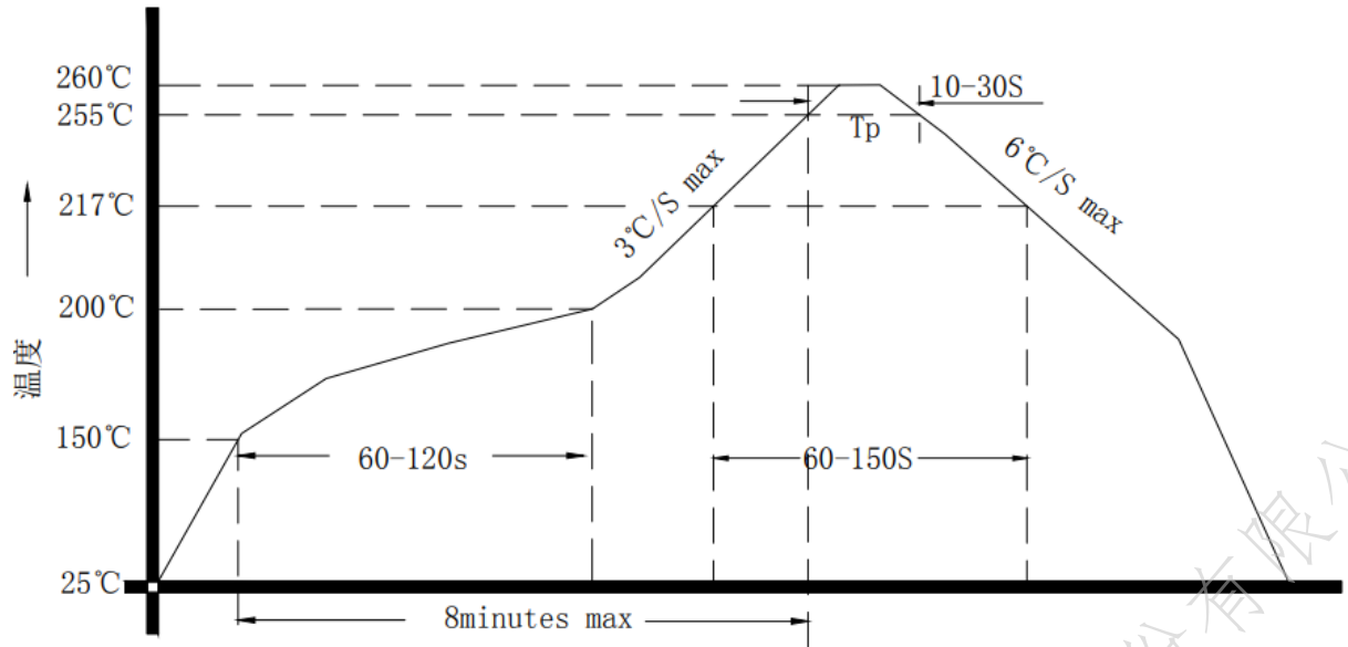
图 3 回流焊曲线
