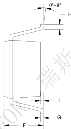
图 4 封装图
