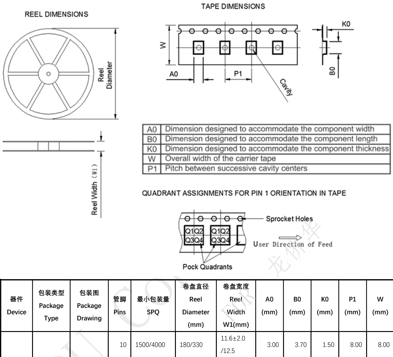
图 6 包装图
