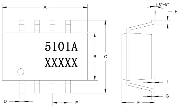
图 4 封装图
