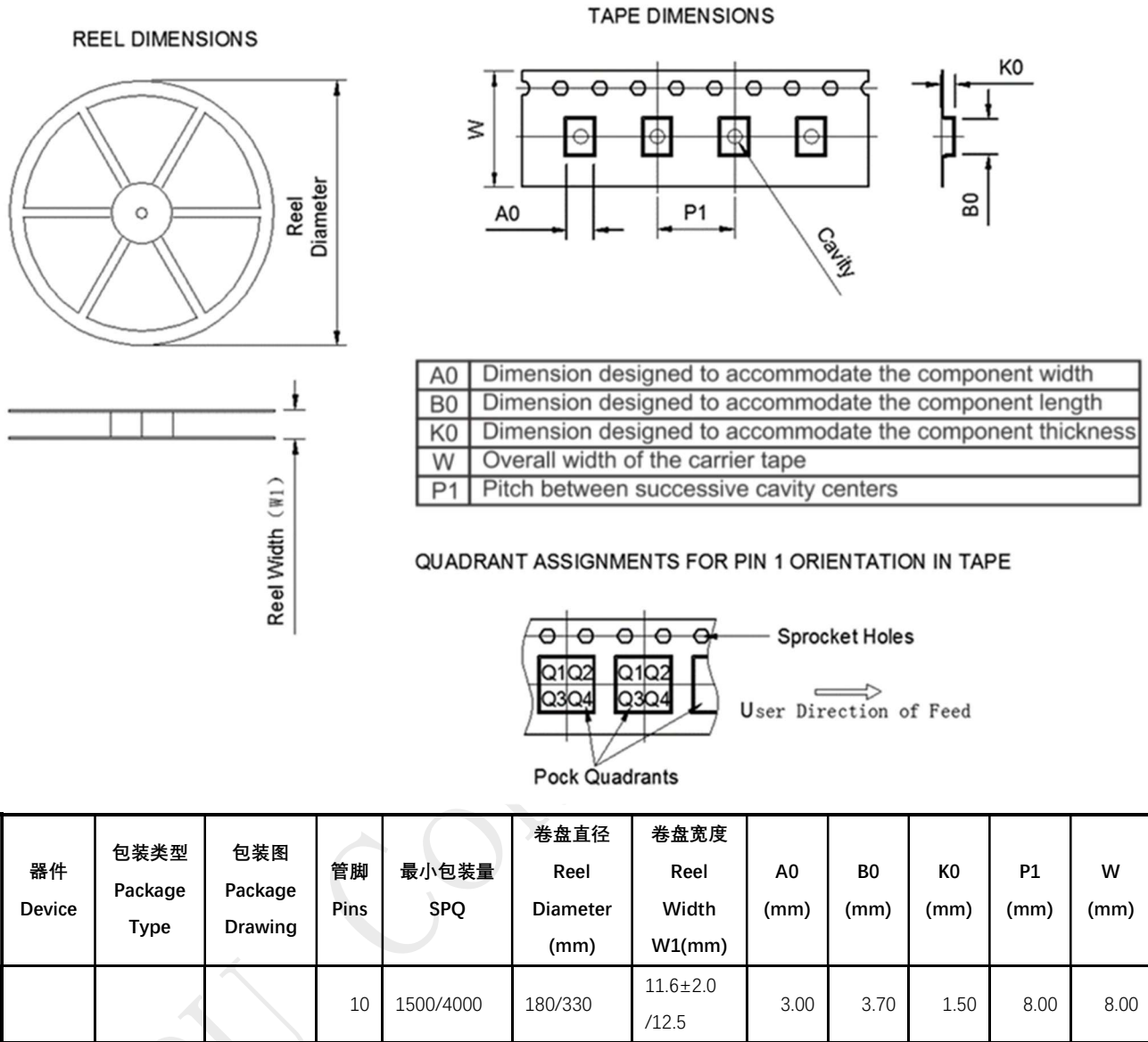
图 5 包装图
