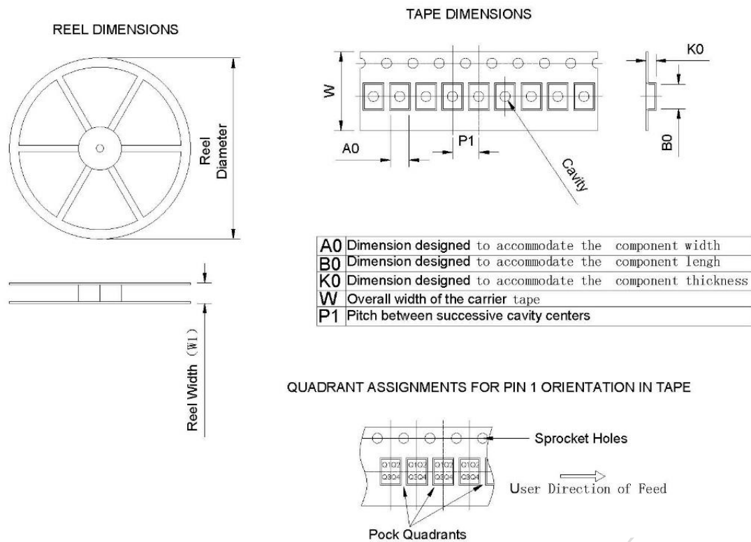
图 11 包装信息
