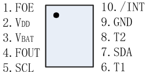
图 2 管脚定义
