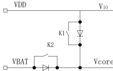
图 4 电源电路框图
