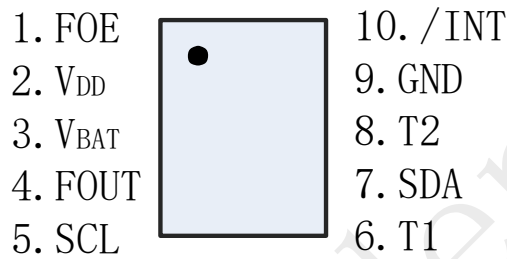
图 2 管脚定义
