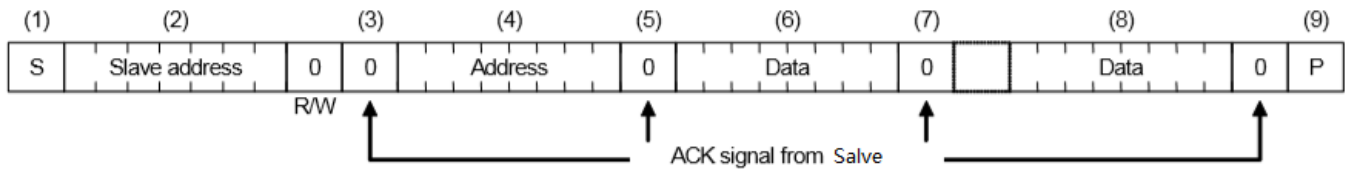
图 6 写序列
