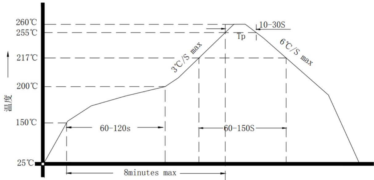
图 10 回流焊曲线
