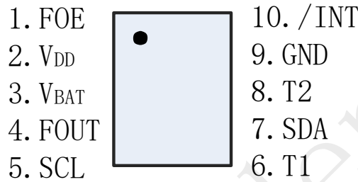
图 2 管脚定义
