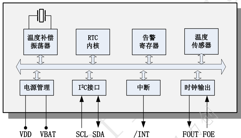
图 1 原理框图
