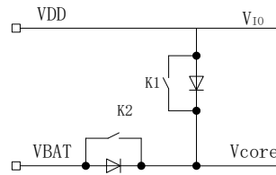
图 4 电源电路框图
