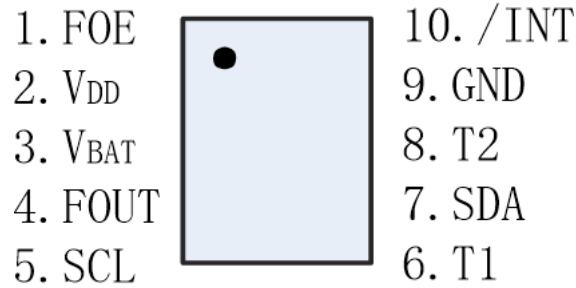
图 2 管脚定义
