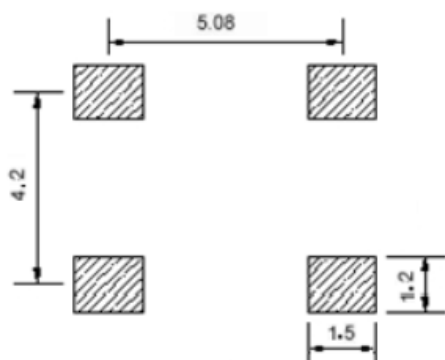
焊盘图
