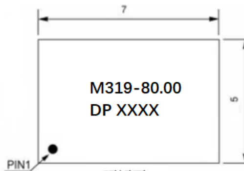
顶视图
