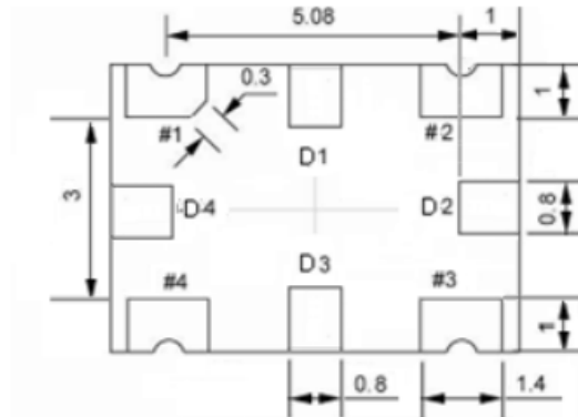
底视图
