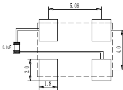
推荐焊盘尺寸 (mm)
